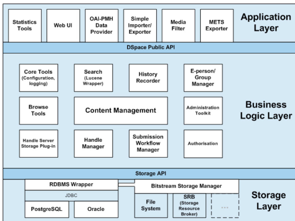
Figura 20: Arquitectura DSPACE
