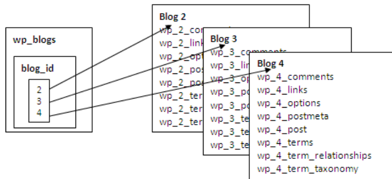
Figura 20. Distribución de blogs internos dentro del Wordpress Multiusuario
